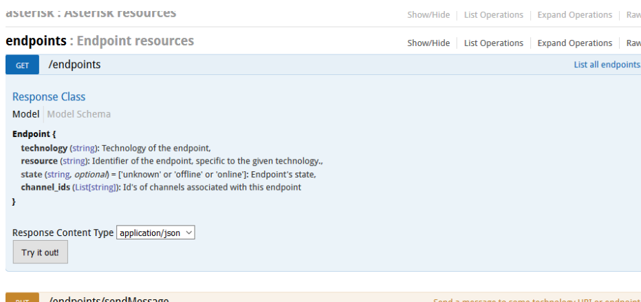
Рисунок 19-3. Получение конечных точек
